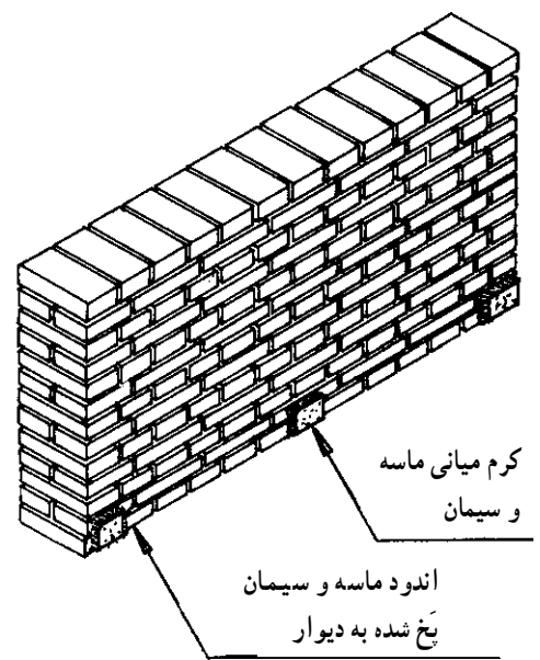
شکل ۲۶-۵- کرم بندی تحتانی به منظور شمشه گیری
