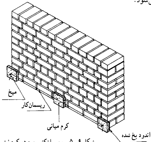
شکل ۹-۵- ریسمان کشی بین دو کرم نش
