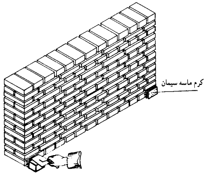
شکل ۲۴-۵- کرم بندی دو نیش دیوار
