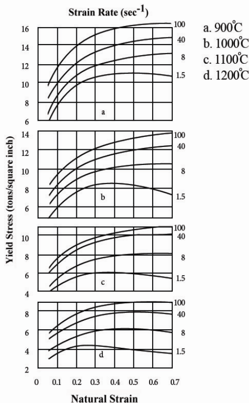
شکل (۳) تنش تسلیم در دماهای مختلف بر حسب کرنش طبیعی برای فولادهای کم کربن [۱۷]
